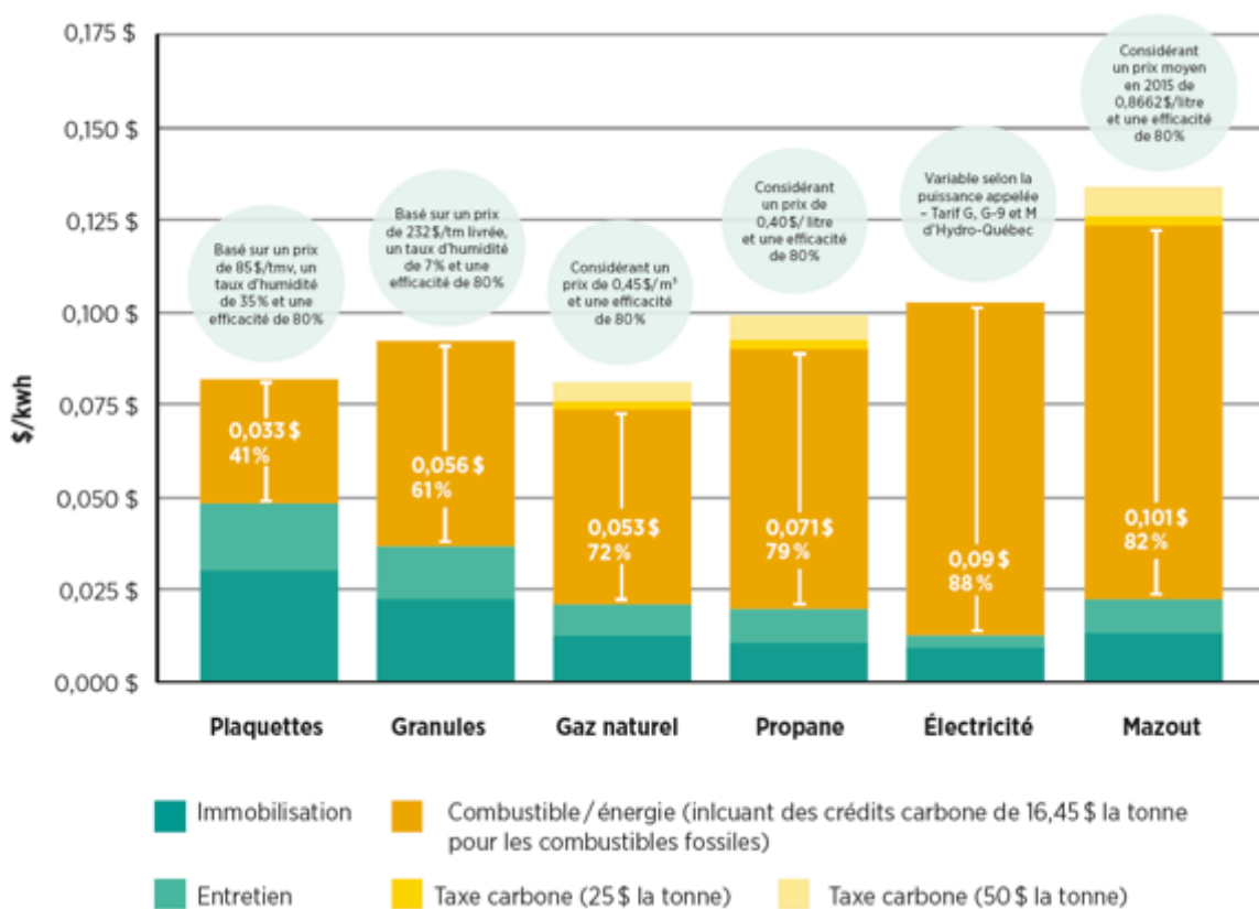
Comparaison des coûts de l'énergie pour la production de chaleur
